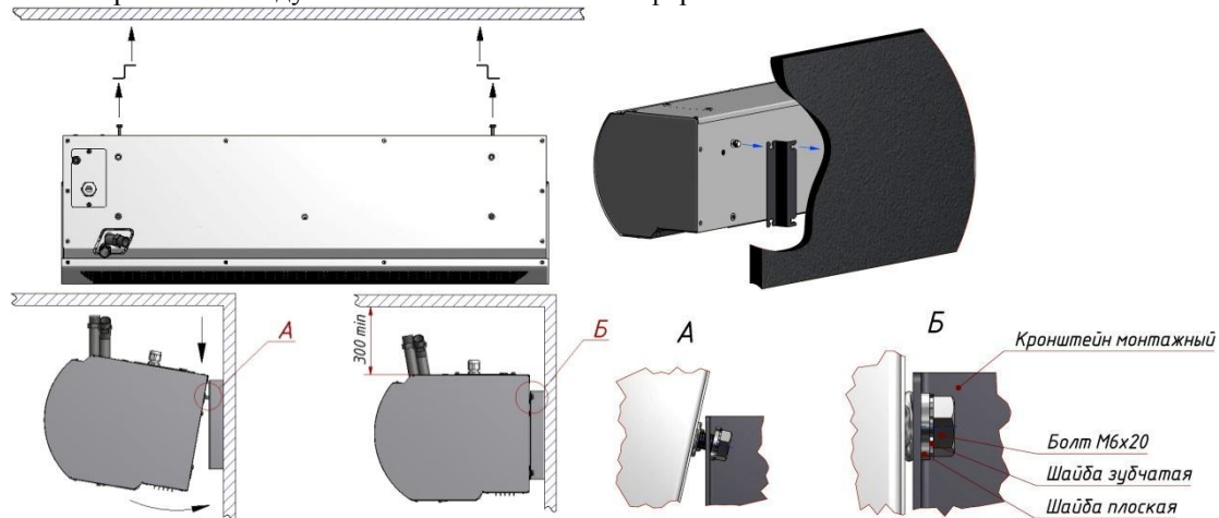
Рисунок 6-Схема крепления воздушно-тепловой завесы «Комфорт»
